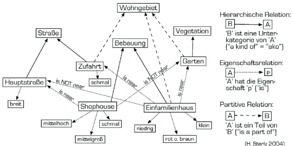
Abbildung 8: Beispiel eines semantischen Netzes, in dem Wissen über die Kategorien „Shophouse“ und „Einfamilienhaus“ repräsentiert ist 44
