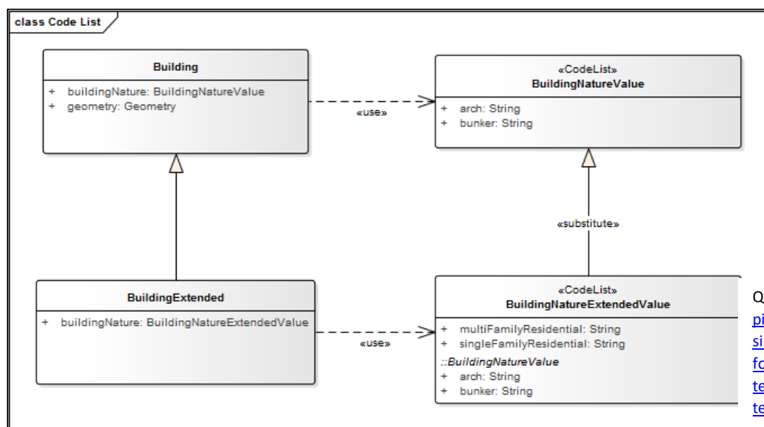
Abbildung 12: Ableitung der erweiterten Codeliste und zusätzliche Ableitung der verwendenden Klasse
