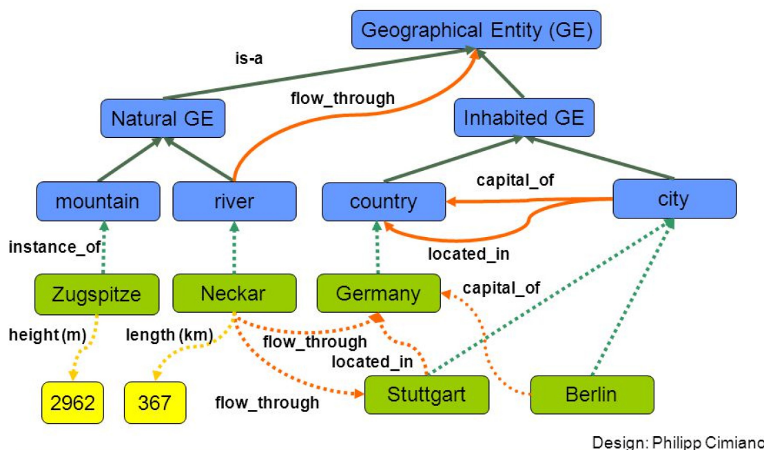
Abbildung 9: Beispiel einer Ontologie zum Thema Geographische Einheiten 46
