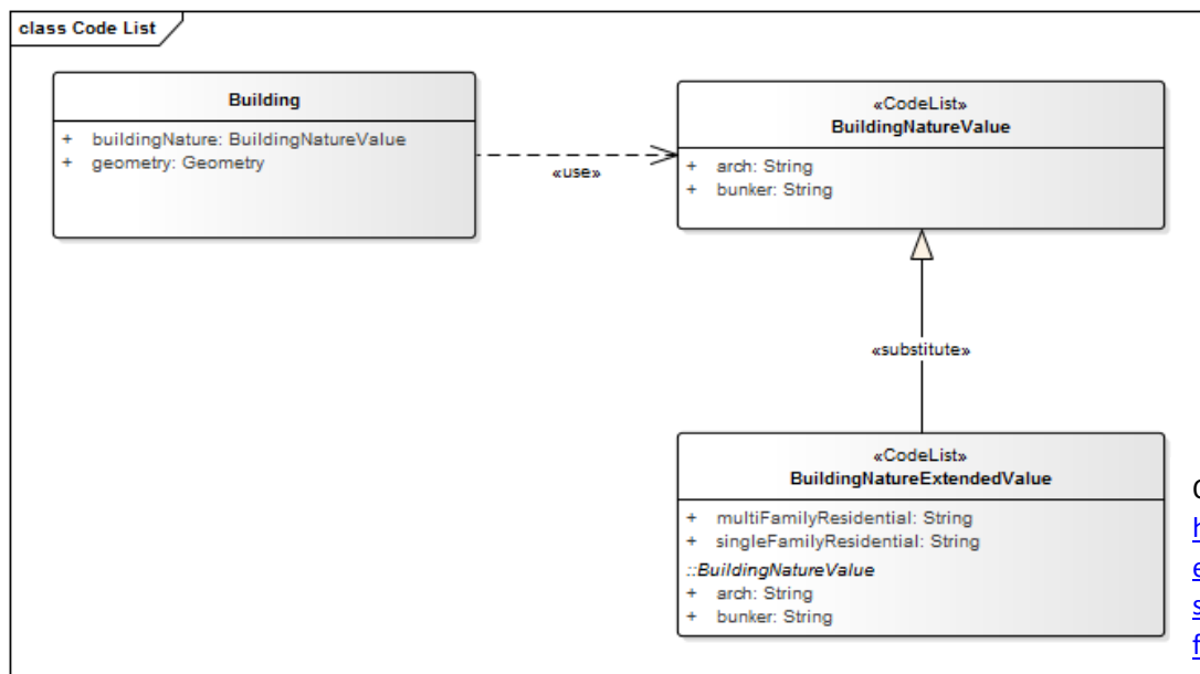
Abbildung 11: Einfache Ableitung der erweiterten Codeliste
