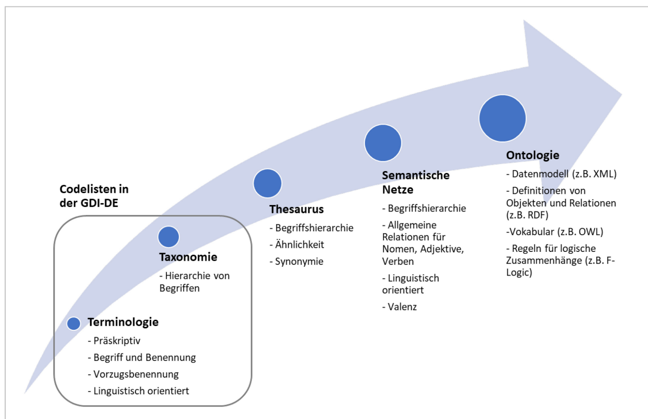
Abbildung 7: Darstellung der verschiedenen mächtigen Systeme der Wissensordnung und -repräsentation (Stichwort: Semantische Treppe nach Blumauer und Pellegrini 42 )
