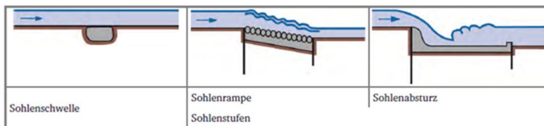
Abbildung 17: Bildliche Darstellung von Bauwerkstypen zur Unterstützung der internationalen semantischen Abstimmung (Quelle DWA 2005)
